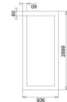
SUPERFICIE APPOGGIO A PAVIMENTO FLOOR SUPPORT AREA
